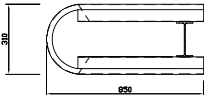
omkeerstuk A/B 008
