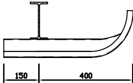
elndstuk A/B 014
