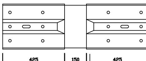
knikplank A/B 016
