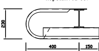
kopstuk A/B 007
